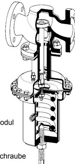
Gehäuse mit Ventil
