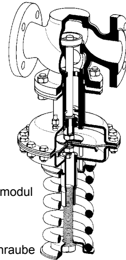
Gehäuse mit Ventil
